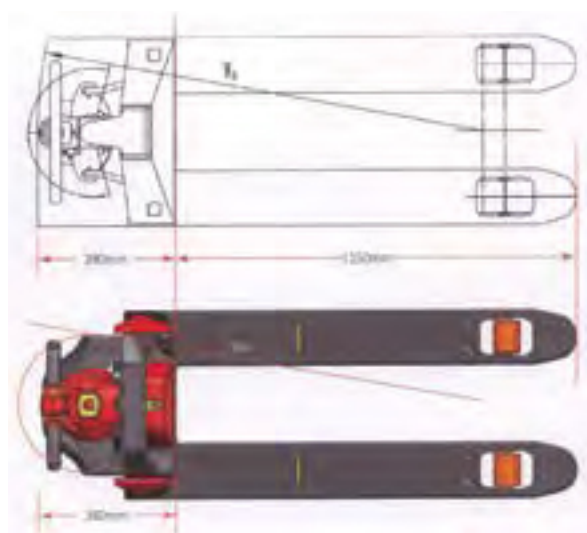
Transpallet manuale
